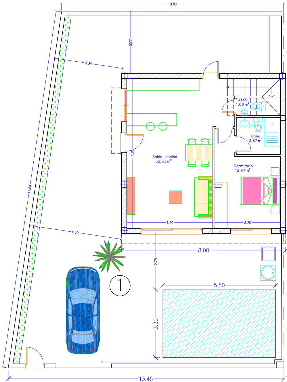
PLANTA 0 Sup. construida=64,40m2
